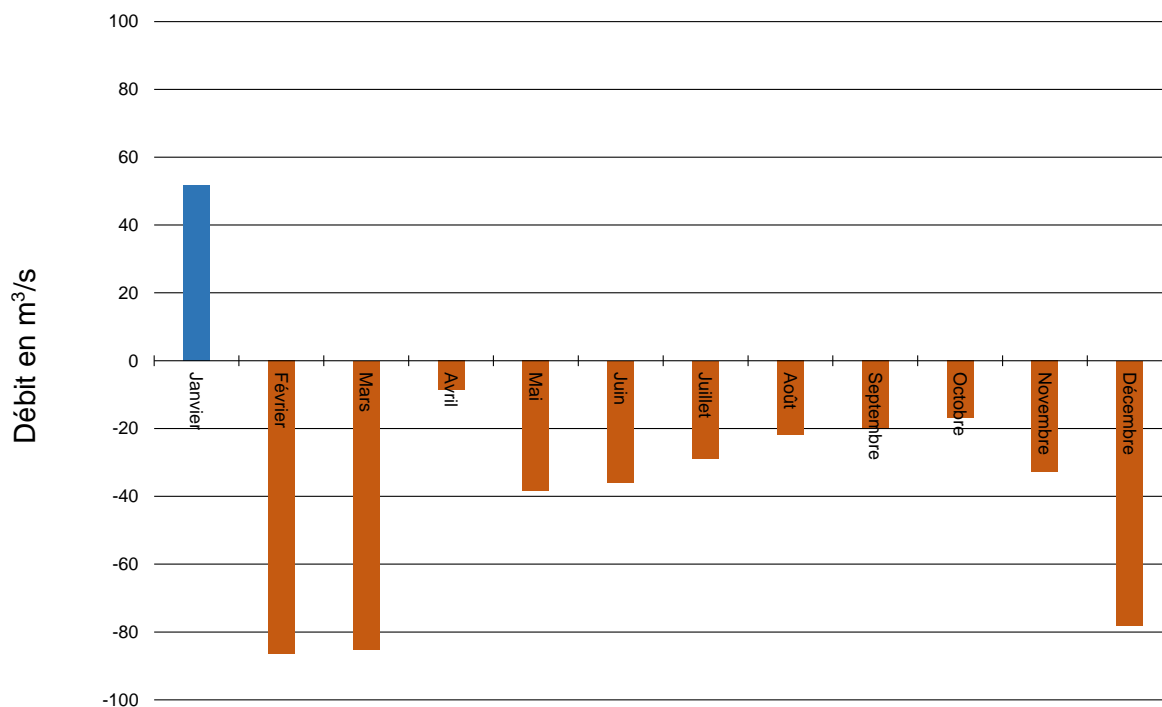
Figure 22 : Différence entre le débit moyen mensuel en 2022 et la moyenne mensuelle interannuelle de 2007-2021
