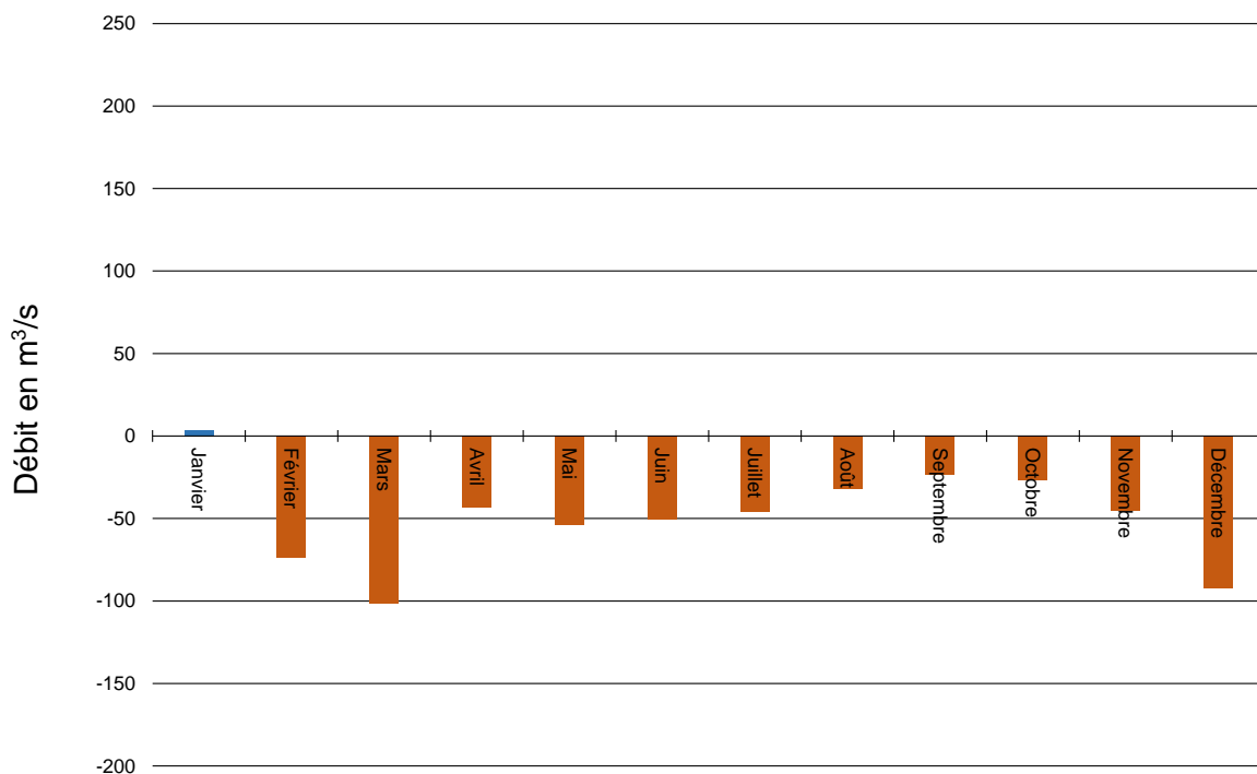
Figure 27 : Différence entre le débit moyen mensuel en 2022 et la moyenne mensuelle interannuelle de 2007-2021
