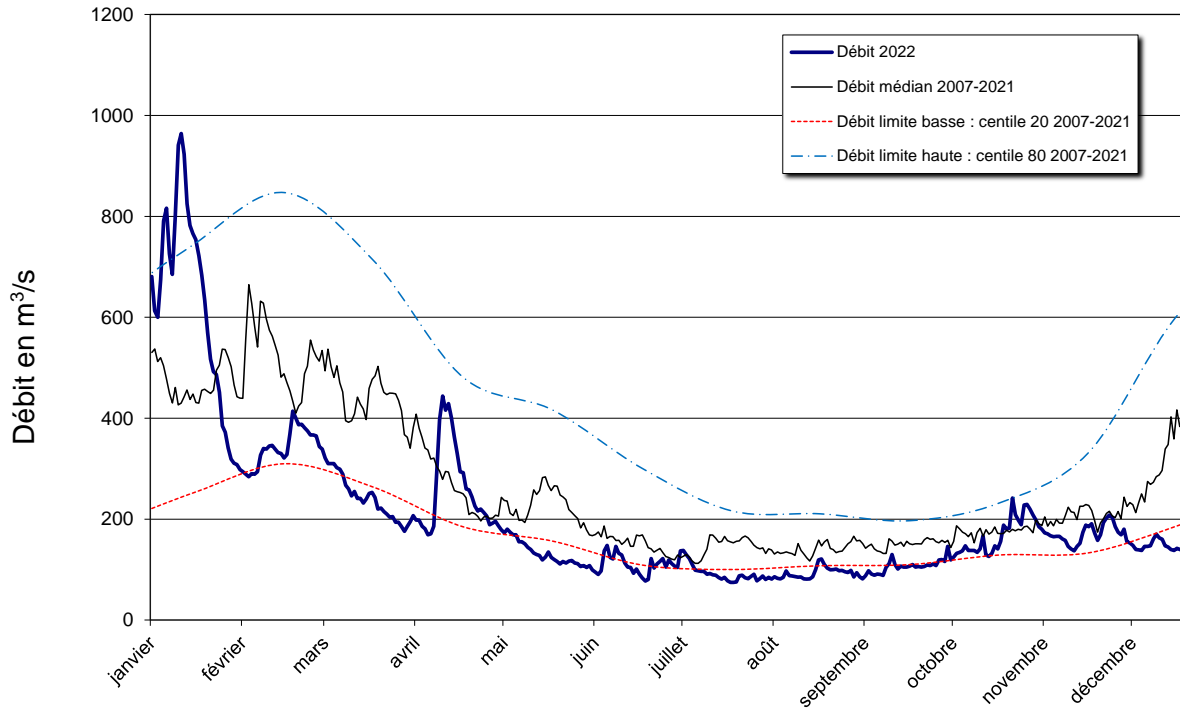
Figure 15 : Débit en Seine en 2022
