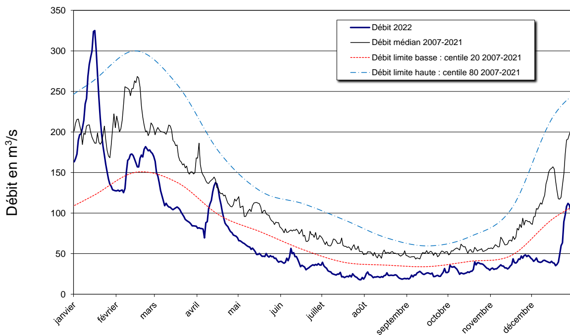
Figure 26 : Débit en Oise en 2022
