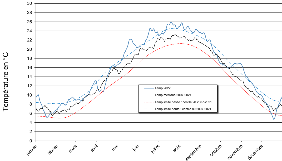
Figure 17 : Température en Seine en 2022
