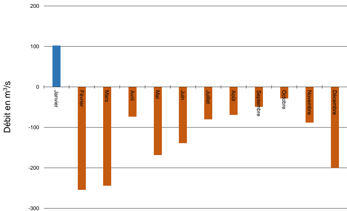
Figure 16 : Différence entre le débit moyen mensuel en 2022 et la moyenne mensuelle interannuelle de 2007-2021
