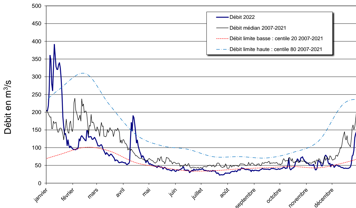
Figure 21 : Débit en Marne en 2022
